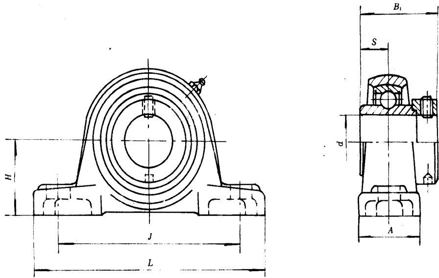
图 2 UELP 型
