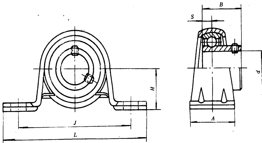
图 18 UBPP 型
