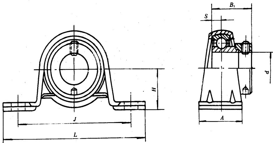
图 19 UEPP 型
