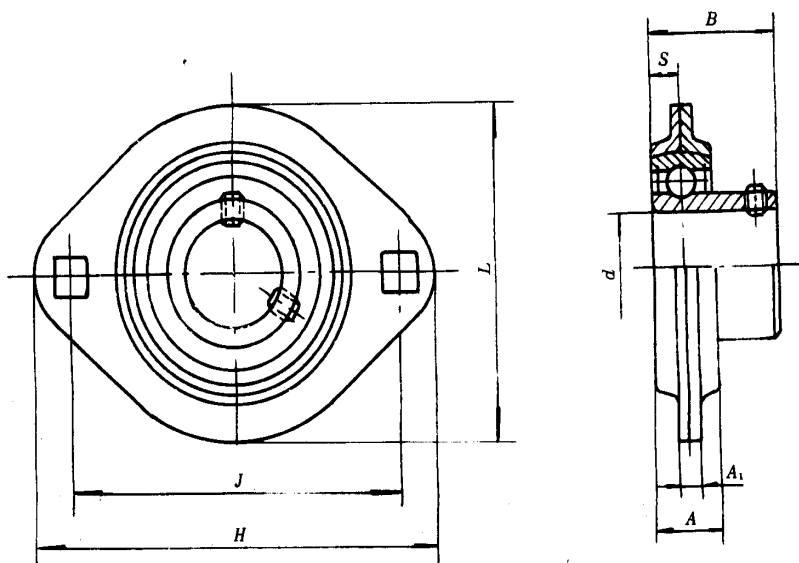
图 24 UBPFL 型
