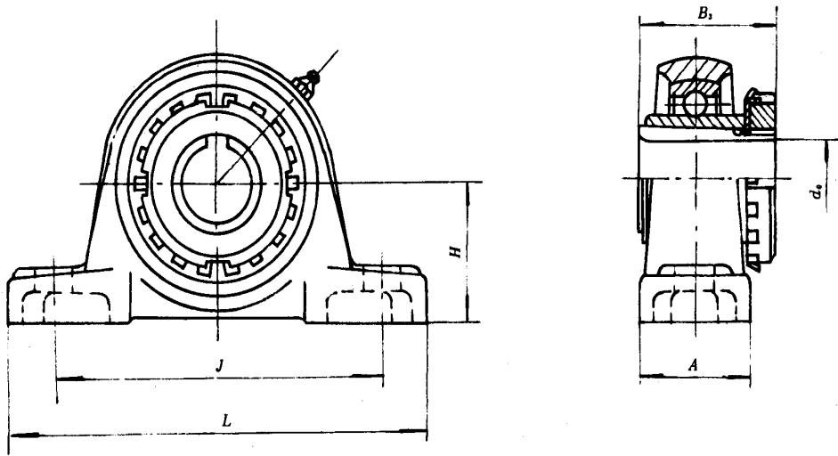
图 3 UKP+H 型
