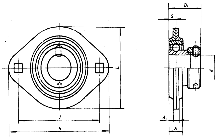
图 25 UEPFL 型
