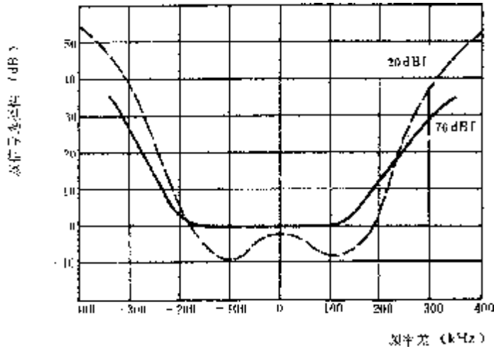
图 21 双信号选择性
