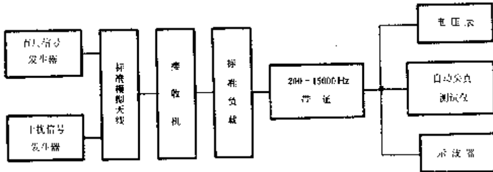
图 20 双信号测试电路
