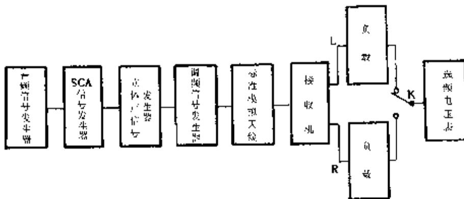
图 53 SCA 抑制测试电路
