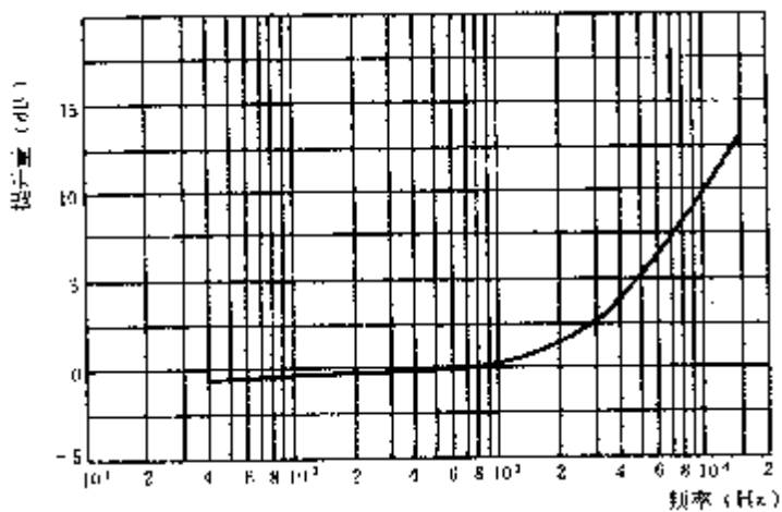
图 8 预加重曲线
