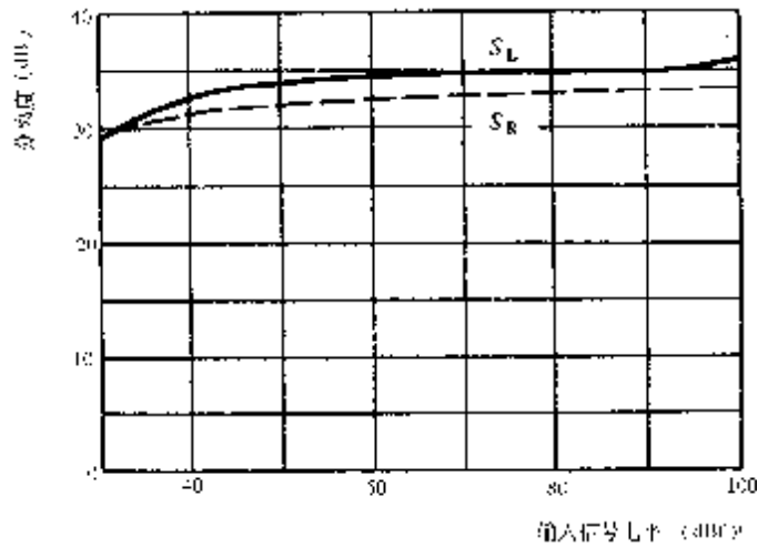
图 49 输入信号电平改变时的分离度 测试频率—98 MHz;调制频率—1 000 Hz; 调制频偏—±20.25 kHz;输出功率—50 mW; 音调—平位
