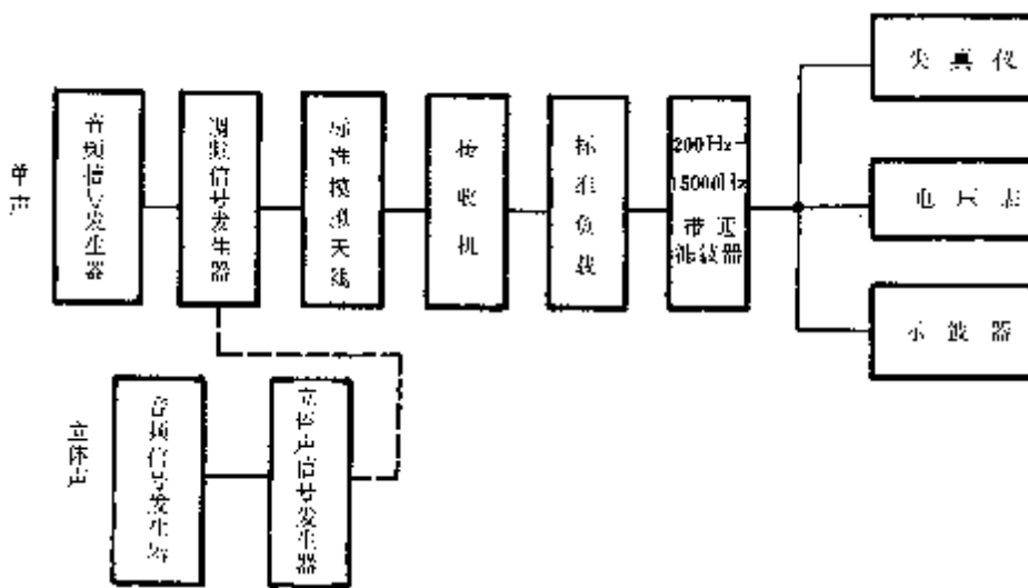
图 30 整机电压谐波失真测试电路
