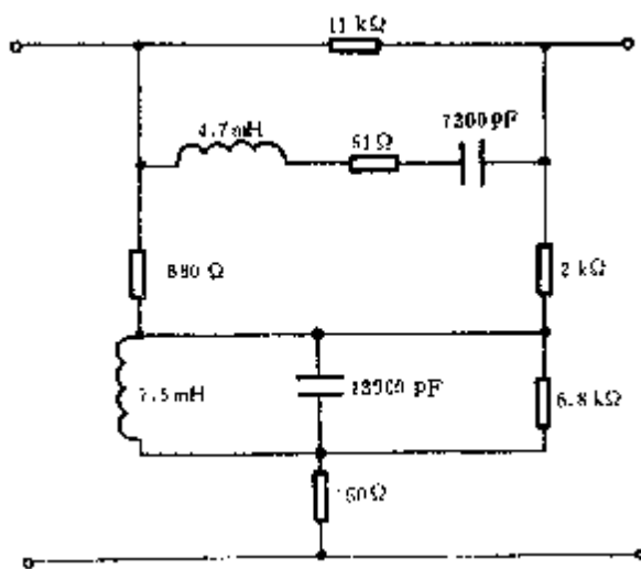
图 9 预加重网络
