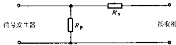
图 3 R_i < R_r 时的单信号标准模拟天线
