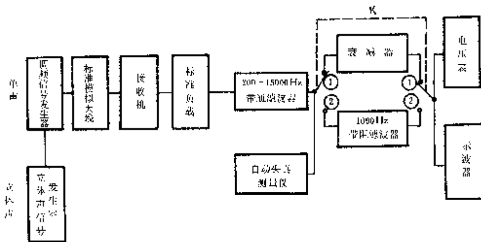
图 15 滤基波法测试电路
