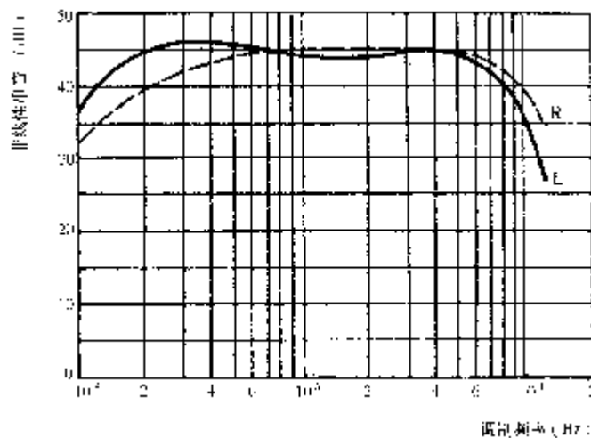
图 50 非线性串音
