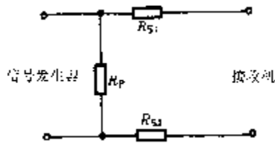
图4 R_i < R_r (平衡) 时的单信号标准模拟天线
