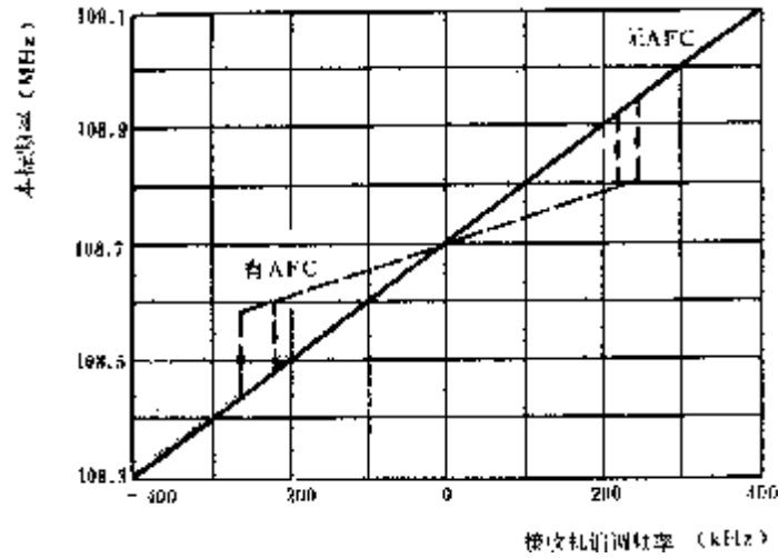
图 44 自动频率控制特性(固定信号发生器频率)
