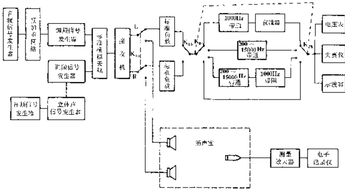
图 10 测试总电路
