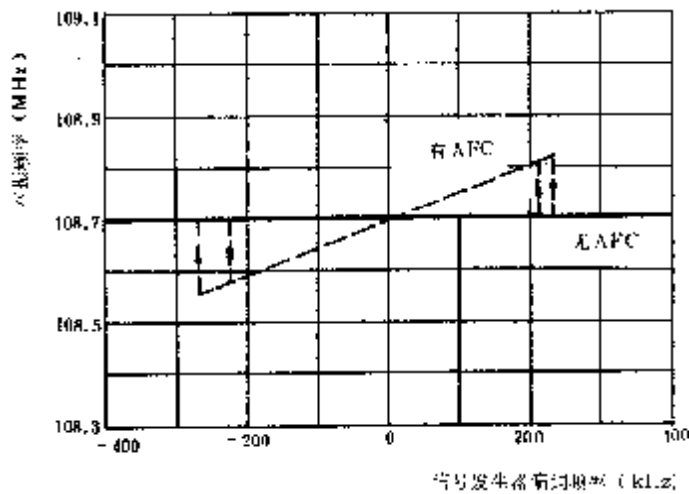
图 45 自动频率控制特性(固定接收机频率)
