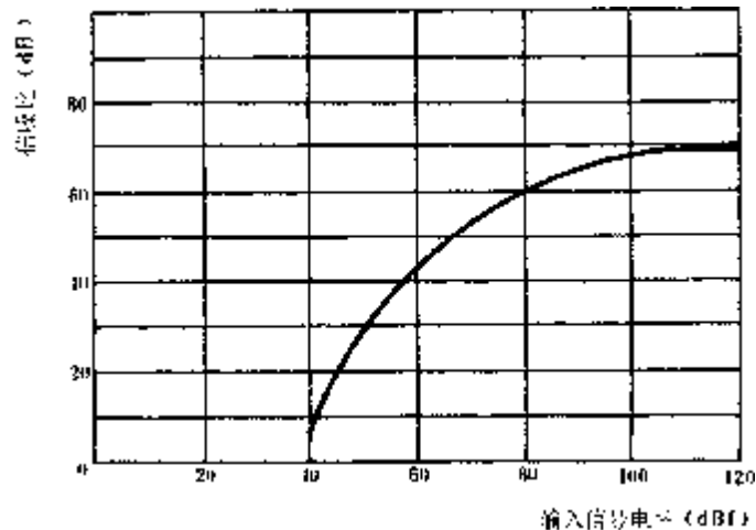
图 46 立体声信噪比(去调制法)
