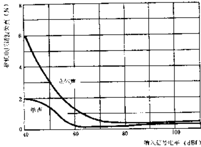
图 33 输入信号电平改变时的失真
