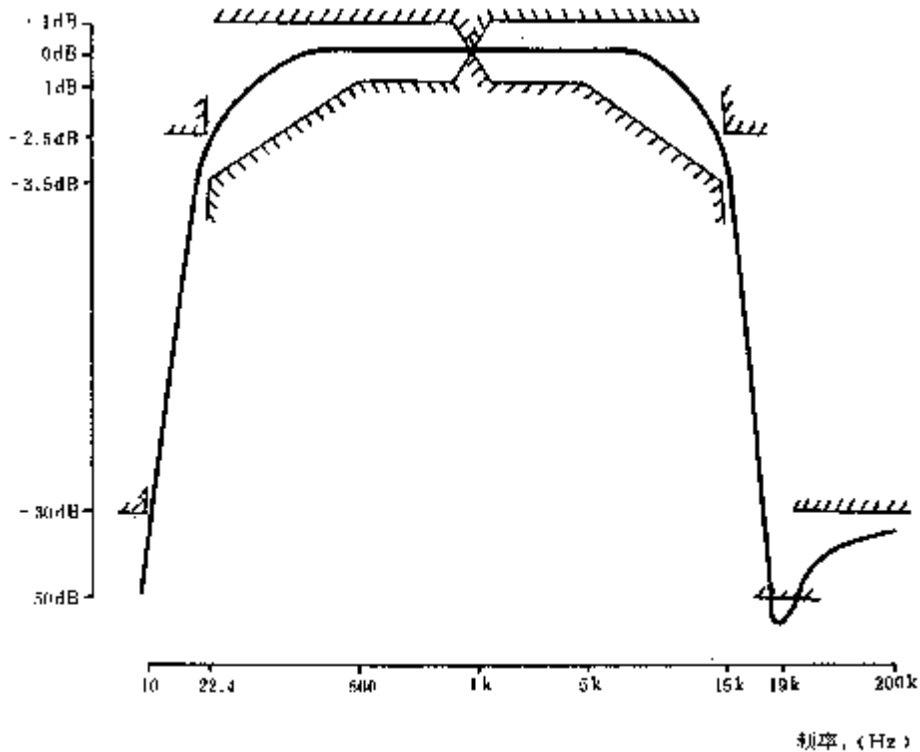
图 12 22.4—15 000 Hz 带通滤波器
