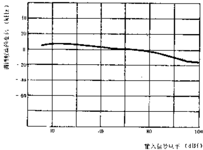
图 43 调谐频率随输入信号电平的变化
