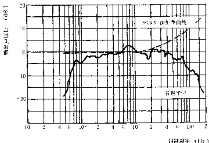
图 38 整机声压频率特性
