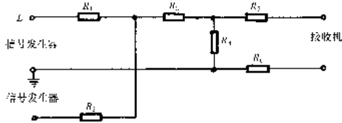
图 7 R_i < R_r (平衡) 时的双信号标准模拟天线
