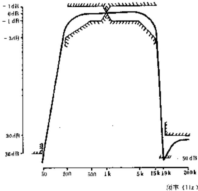
图 11 200—15 000 Hz 带通滤波器
