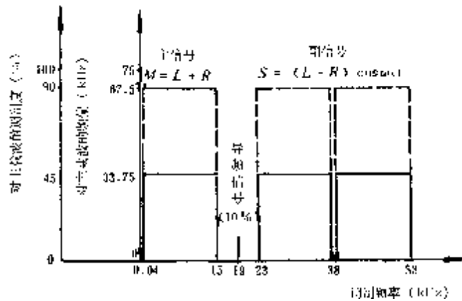
图 1 立体声复合信号的频谱图
