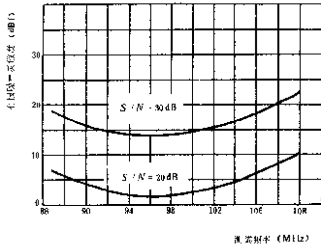
图 16 有限噪声灵敏度 调制频率—1 000 Hz;频偏— \pm 75 kHz; 输出功率—50 mW;音调—窄位
