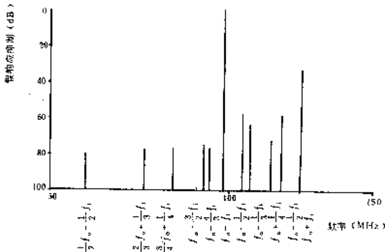
图 25 单信号假响应(已调信号法) 测试频率—98 MHz;调制频率—1 000 Hz;输入 信号电平—限幅灵敏度;频偏—±22.5 kHz; 输出功率—50 mW;音调—平位
