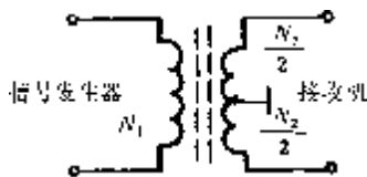
图5 采用平衡-不平衡变换器的标准模拟天线
