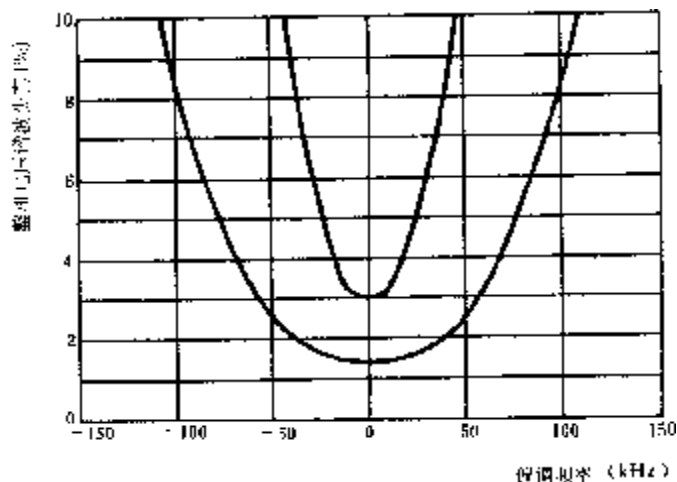
图 35 偏调失真
