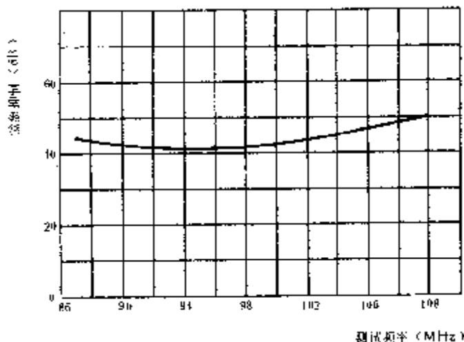
图 24 单信号镜象抑制 调制频率—1 000 Hz;频偏—±22.5 kHz; 输入信号电平—限幅灵敏度;输出 功率—50 mW;音调—平位
