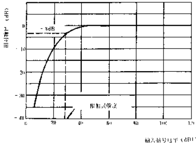
图 18 限幅灵敏度
