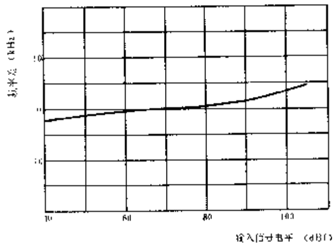
图 39 调谐指示的准确度 测试频率—98 MHz; 调制频率—1 000 Hz; 输出功率—50 mW
