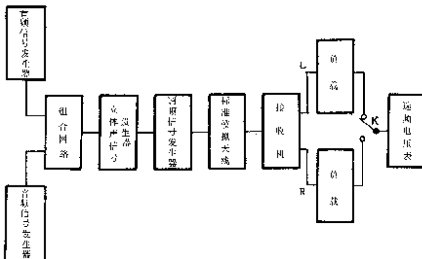
图 52 通道内互调的测试电路
