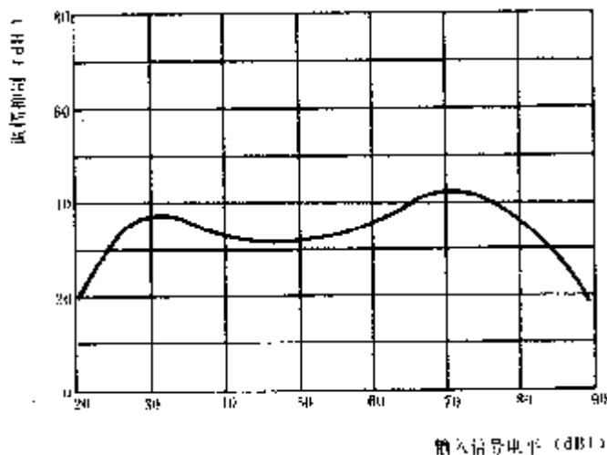
图 27 调幅抑制(同时调制法)
