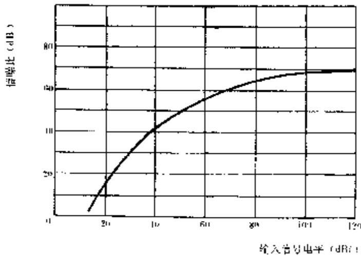
图 14 信噪比(去调制法)
