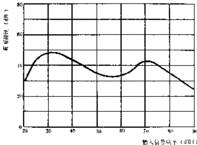
图 28 调幅抑制(顺序调制法) 测试频率—98 MHz;调制频率—1 000 Hz; FM 频偏—±75 kHz;AM 调制度—30%; 输出功率—50 mW;音调—平位
