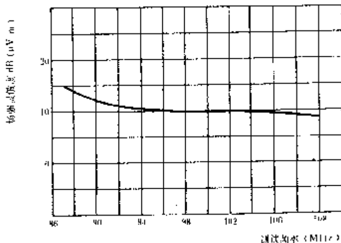
图 17 机内天线接收机的场强灵敏度
