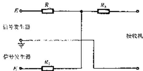
图6 R_i = R_r 时的双信号标准模拟天线
