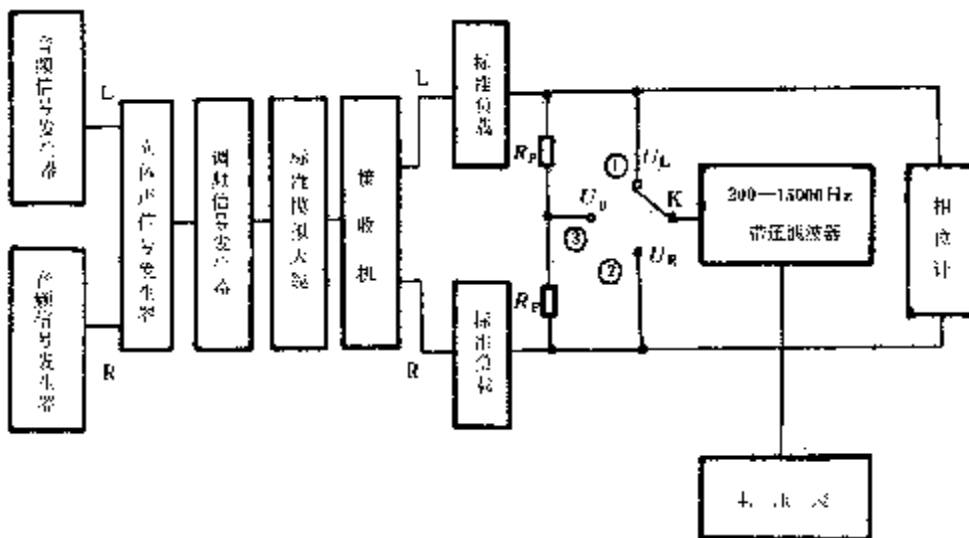
图 47 立体声性能的测试电路 R P 为平衡电阻，接收机 R P =1 kΩ； 调谐器 R P =1 MΩ
