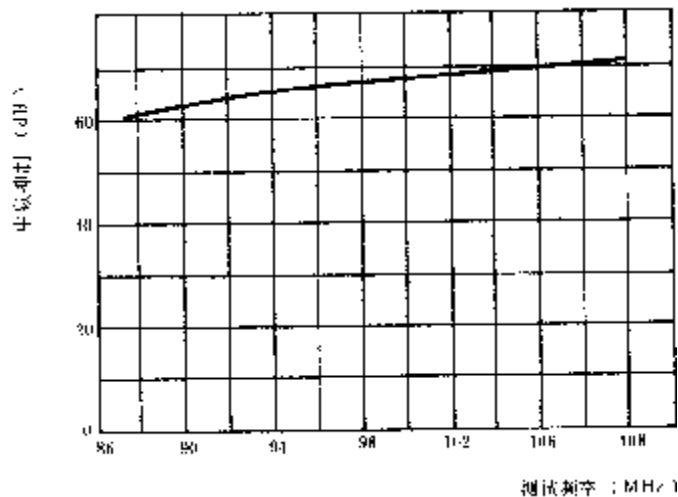
图 23 中频抑制
