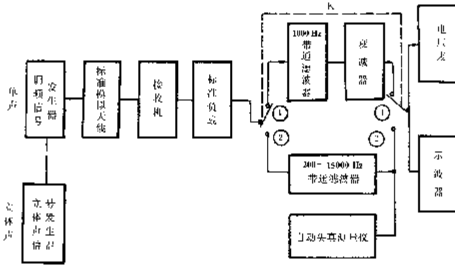
图 13 去调制法测试电路
