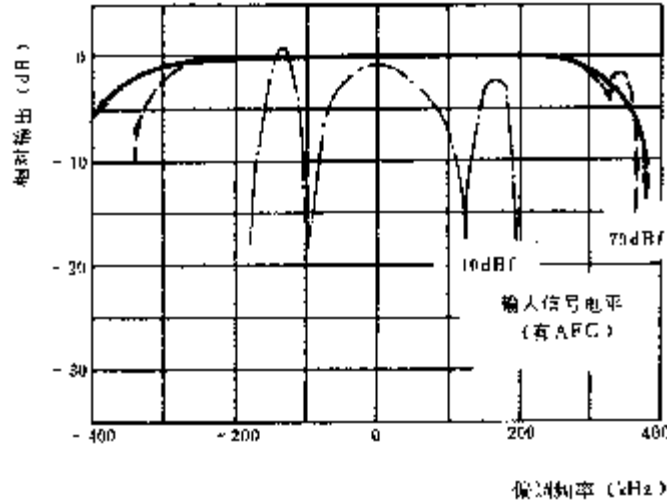
图 29 调谐特性
