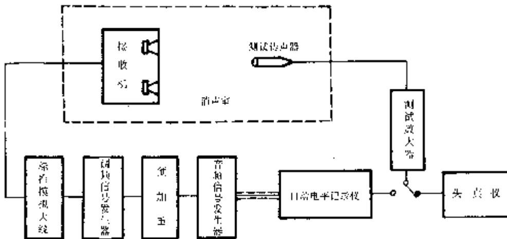
图 36 整机声性能测试电路
