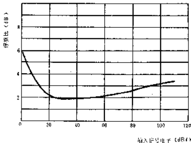
图 26 俘获比
