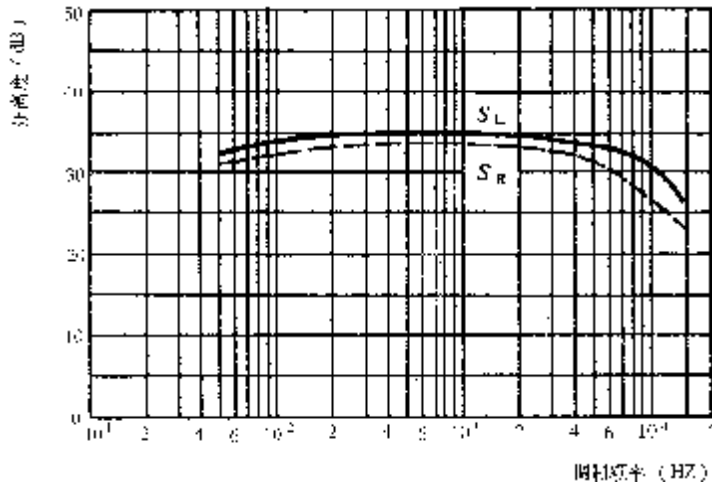
图 48 调制频率改变时的分离度 测试频率—98 MHz;频偏—±20.25 kHz; 输入信号电平—70 dBf;输出功率—50 mW; 音调—平位
