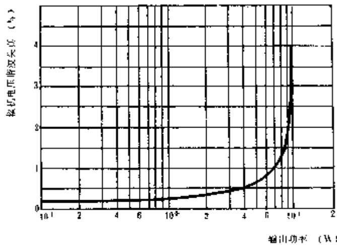
图 34 输出功率改变时的失真
